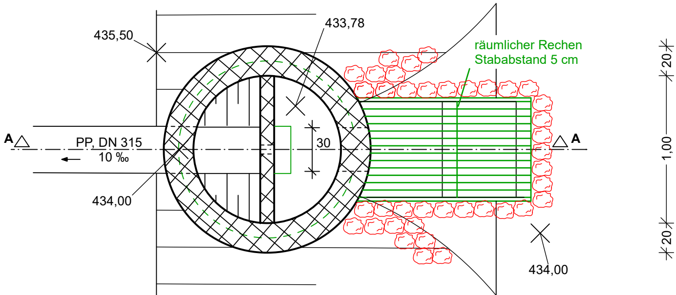
Grundriss
